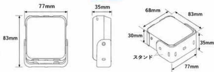
寸法図
